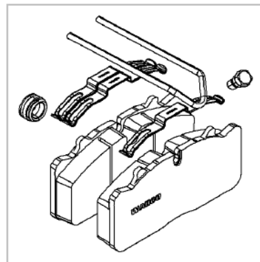
Obr. 1: Opravárenská sada WABCO
