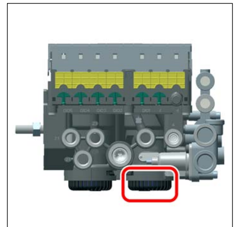
Modulátor pro Trailer EBS-E s místem možného úniku vzduchu
